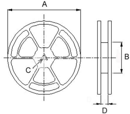
Reel Dimensions
