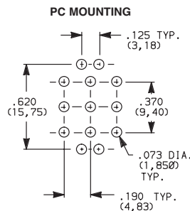
7301J1_BE2 3PDT
