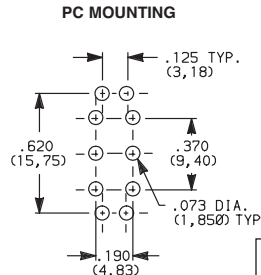
7201J1_BE2 DPDT
