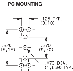
7101J1_BE2 SPDT
