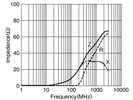
MMZ1608D800C
