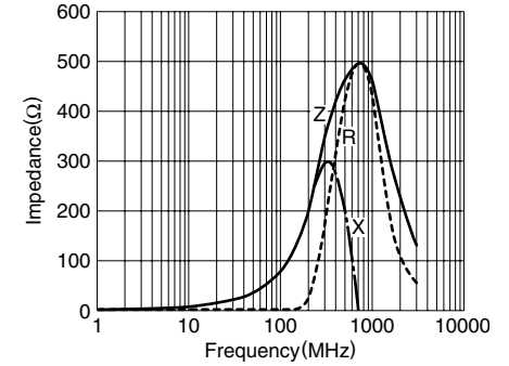
MMZ1608D800C
