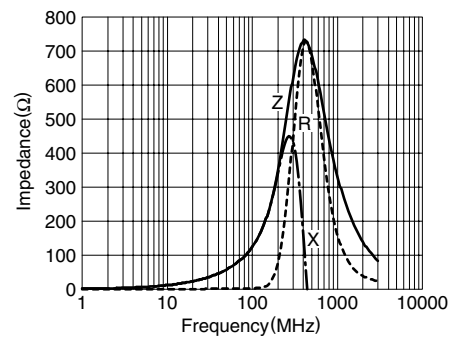
MMZ1608D121B
