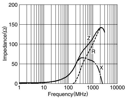
MMZ1608D220C
